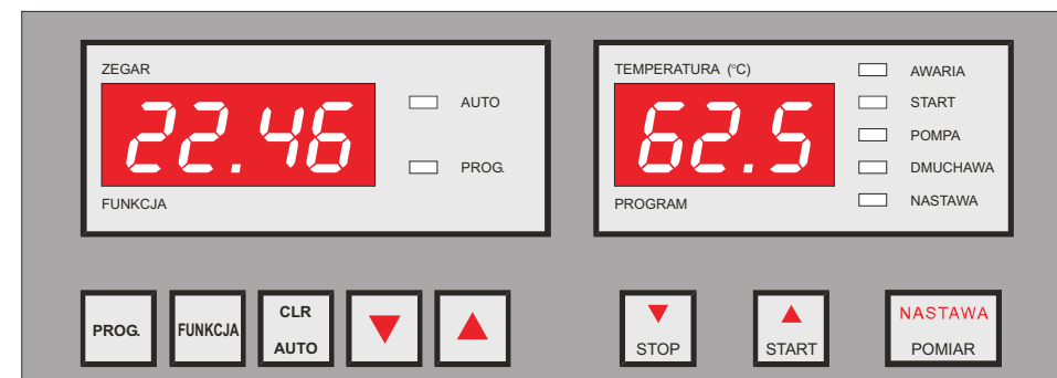
Widok panelu sterowania z przyciskami sterującymi.
