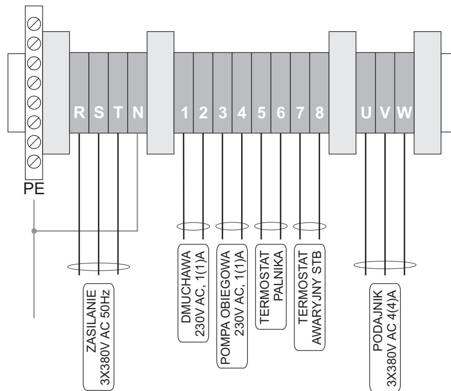
Widok listwy zaciskowej.
