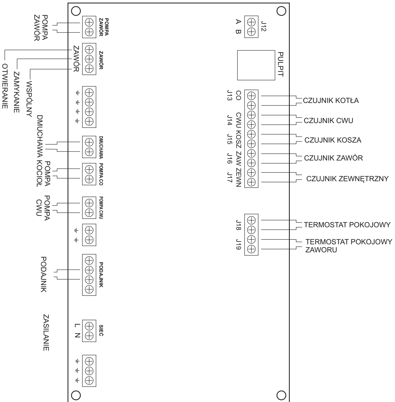
Rys.19. Widok płyty głównej z kostkami montażowymi do podłączenia urządzeń wejścia/wyjścia.
