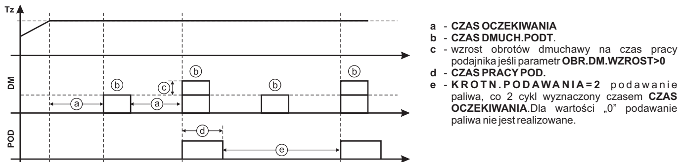
Rys.12. Interpretacja graficzna sposób działania podajnika i dmuchawy.
