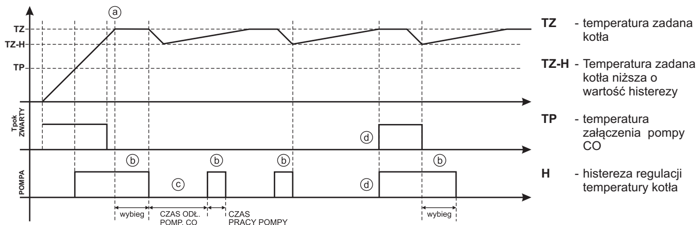
Rys.10. Zmiany temperatury na kotle i zachowanie urządzeń dla ALGORYTM=2
