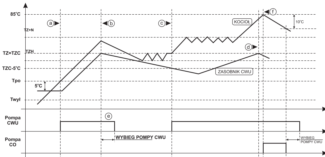
Rys.14. Wykres pracy pompy CO i pompy CWU dla TRYB PRACY CWU=LATO.
