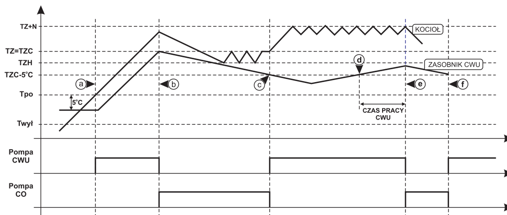
Rys.13. Wykres pracy pompy CO i pompy CWU dla TRYB PRACY CWU=ZIMA i PRIORYTET=WŁĄCZONY .
