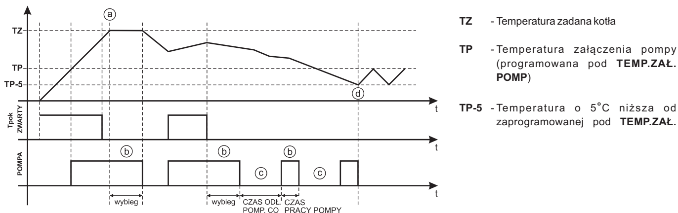
Rys.9. Zachowanie modułu i przebieg temperatury na kotle dla ALGORYTM=0
