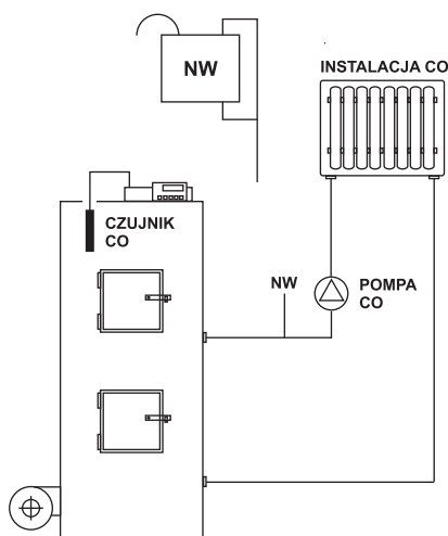
Rys.1. Schemat instalacji kotła nadmuchowego z jednym obiegiem grzewczym
